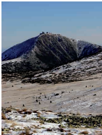
Ryc. 12. Szczyt Śnieżki zbudowany jest ze skał odpornych na wietrzenie – hornfelsów. Jej kształt związany jest z działalnością zlokalizowanych u jej podnóża przed tysiącami lat lodowców
