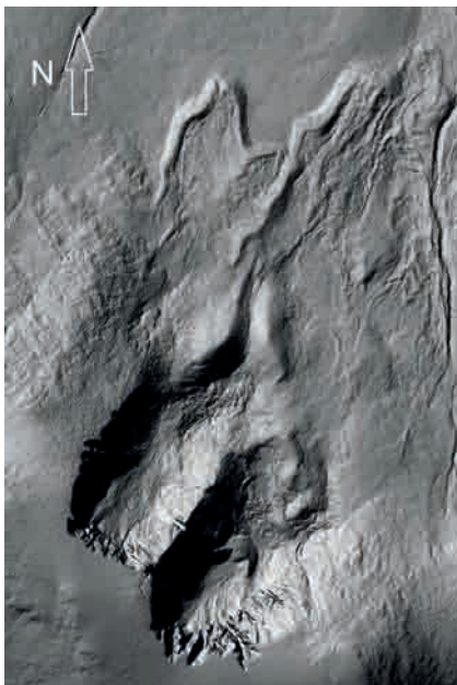
Ryc. 69. Zasięg moren lodowca Śnieżnych Kotłów doskonale prezentuje się na trójwymiarowym modelu rzeźby Karkonoszy
