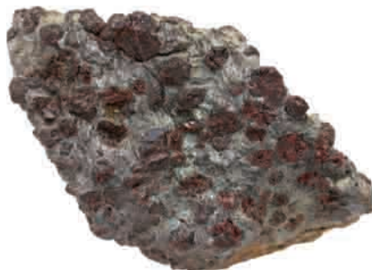
Ryc. 137. Łupek łuszczykowy z granatami z Sowiej Doliny
