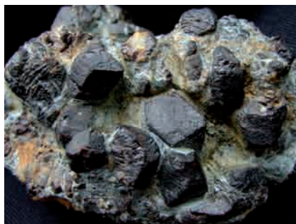
Ryc. 142. Prawidłowo wykształcone kryształy granatów ze Skalnego Stołu
