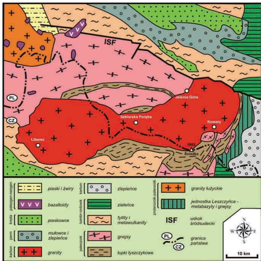
Ryc. 5. Mapa geologiczna Karkonoszy i okolic
