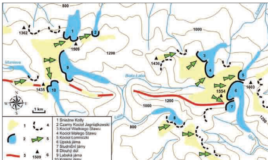
Ryc. 16. Maksymalny zasięg lodowców w epoce lodowej w Karkonoszach polskich i czeskich: 1- powierzchnia zrównania wierzcholinowego, 2- krawędzie kotłów z maksymalnym zasięgiem lodowców górskich, 3- hornfelsowy grzbiet, 4- strefy ze słabo wykształconą rzeźbą polodowcową (nisze niwalne), 5- kierunki przewiewania śniegu z wierzchliny, 6- ważniejsze szczyty (wg P. Migonia)
