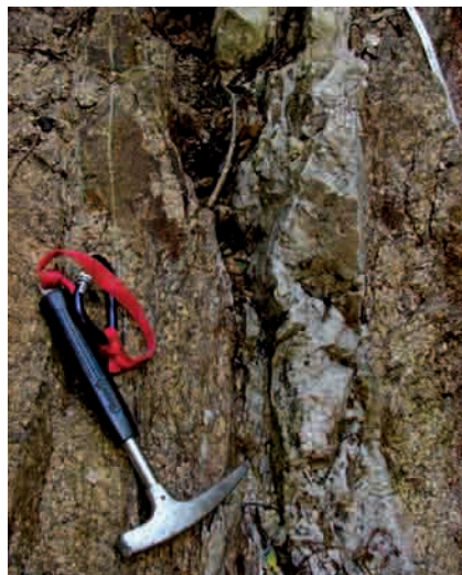
Ryc. 42. Żyła kwarcu mlecznego odslaniająca się w Wąwozie Kamieńczyka
