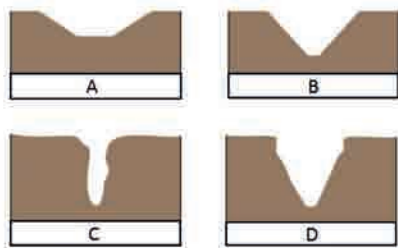
Ryc. 37. Typy dolin rzecznych: A – płaskodenna, B – wcięta, C – gardziel, D – jar
