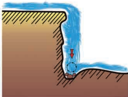
Ryc. 44. Schemat ilustrujący powstawanie kotłów eworsyjnych u progu wodospadu
