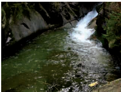
Ryc. 45. Szeroki kocioł eworsyjny u podnóża Wodospadu Szklarki
